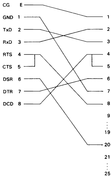
Fig. 4.16 Cable #725
